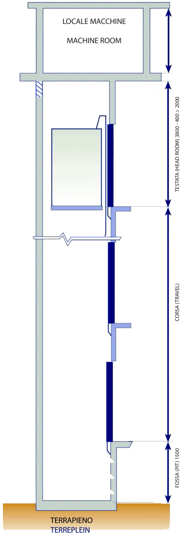
SEZIONE VANO CORSA E LOCALE MACCHINE SHAFT AND MACHINE ROOM SECTION
